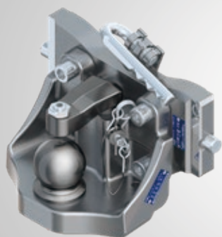
80mm 球头装置 (舒适型)
